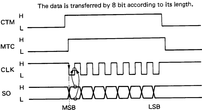
Fig. 12 Timming chart
