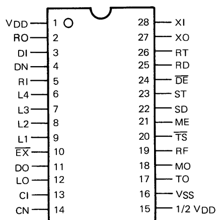
Fig. 14 MN6127A (DCL unit IC2)
